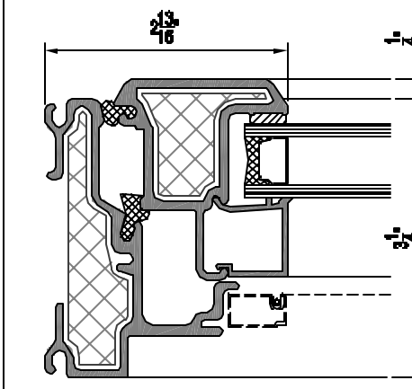
3 JAMB DETAIL 325
